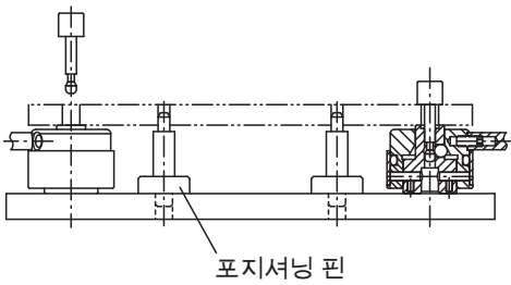
텐션 클램프와 텐션 핀을 이용한 클램핑
