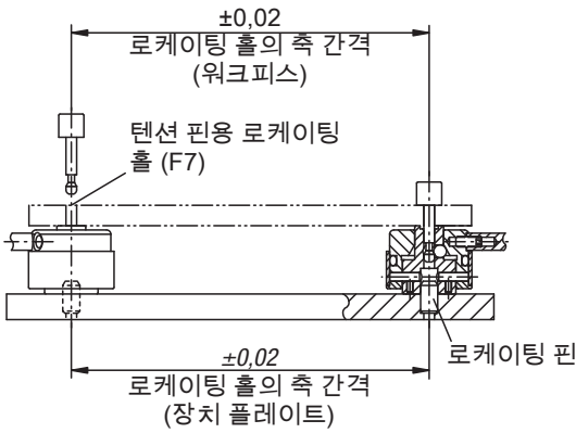
워크피스의 클램핑과 포지셔닝 동시 실행
