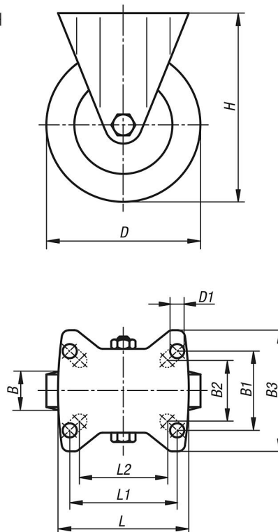
고정 캐스터
