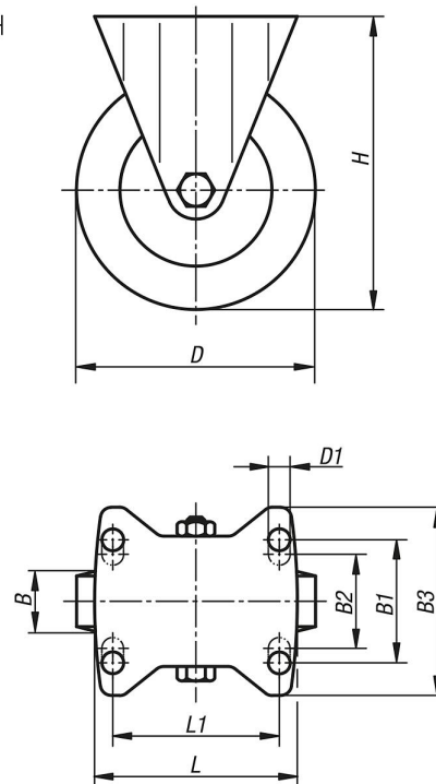
고정 캐스터
