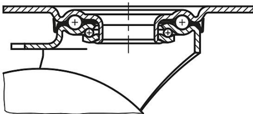
턴테이블 베어링, R1 = 125까지
