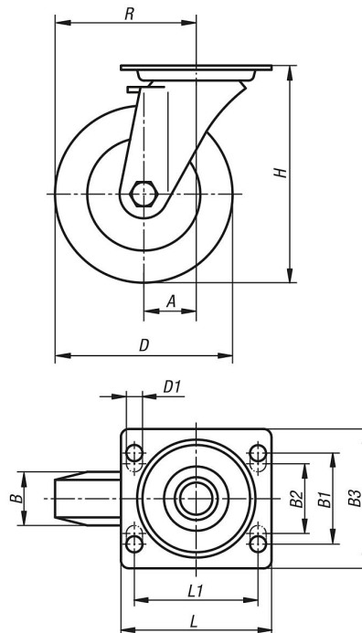
스위벨 캐스터
