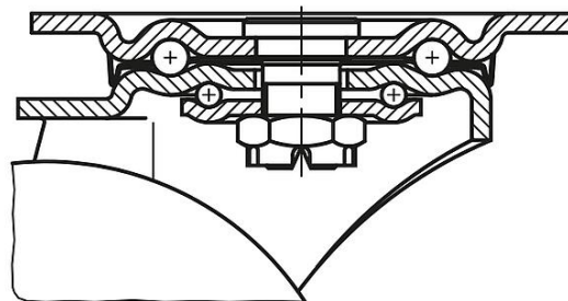
턴테이블 베어링, R1 = 160부터
