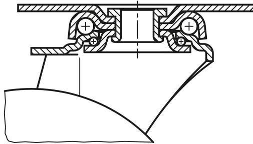
턴테이블 베어링:
