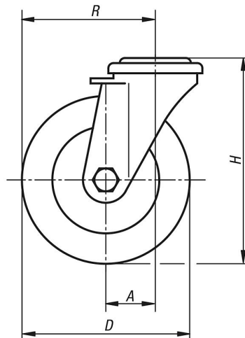
스위벨 캐스터
