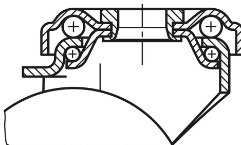
턴테이블 베어링:
