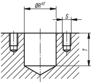
마운팅 홀의 치수
