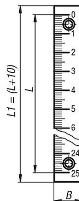
홀 있음 조립 위치, 수직
